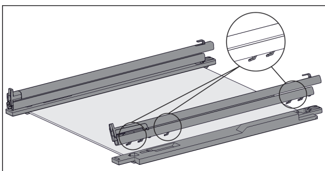
Fig. 59 Скляна пластина з рейками та деталями для підтримки
